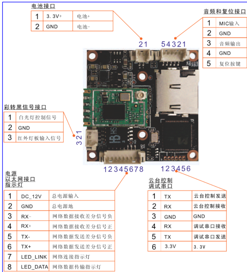
图 1.2 主板背面图
