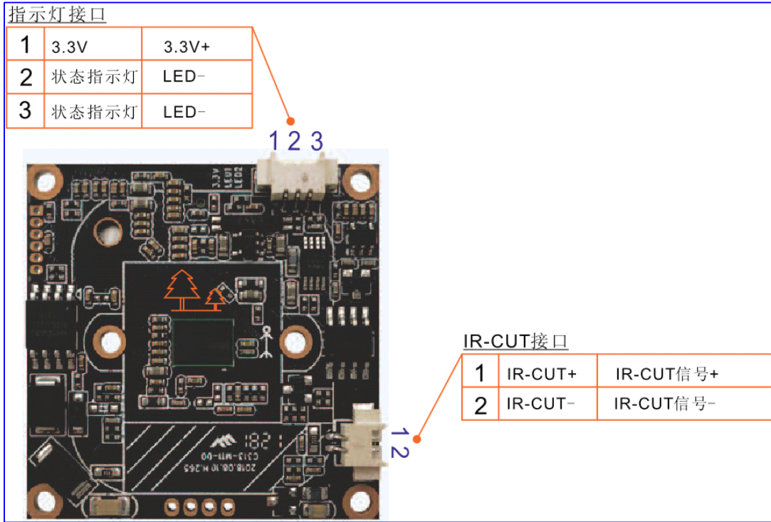
图 1.1 主板正面图
